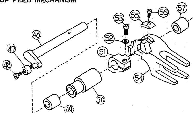
上送り機構 TOP FEED MECHANISM
