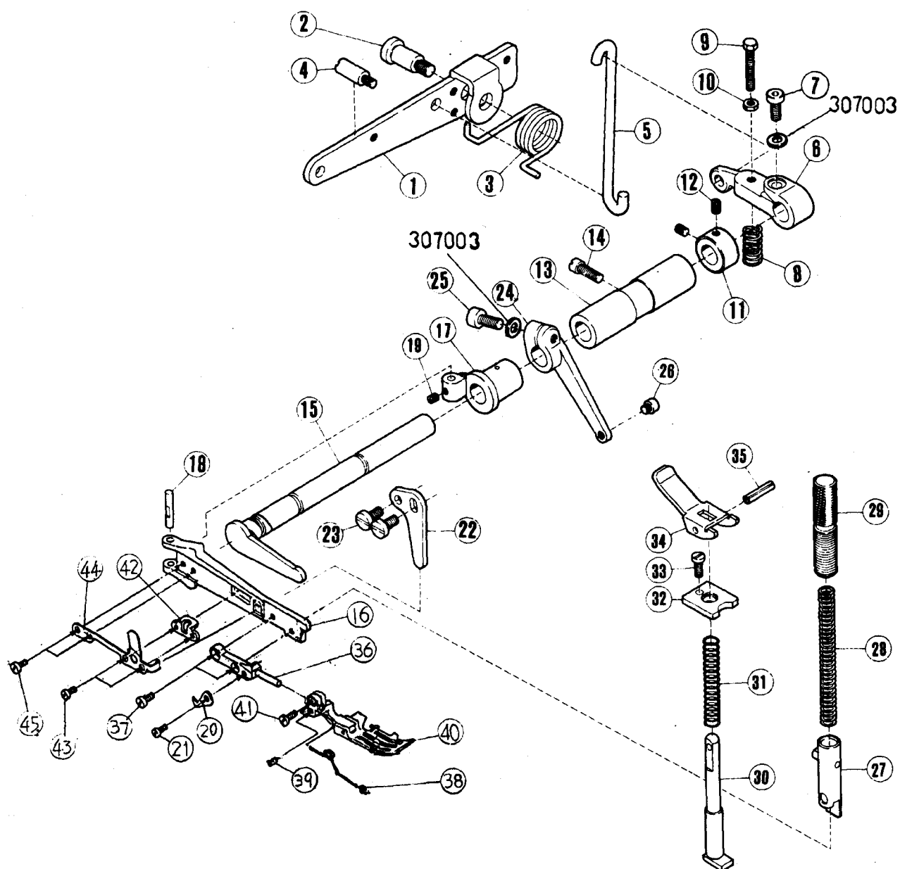
上送り機構 TOP FEED MECHANISM
